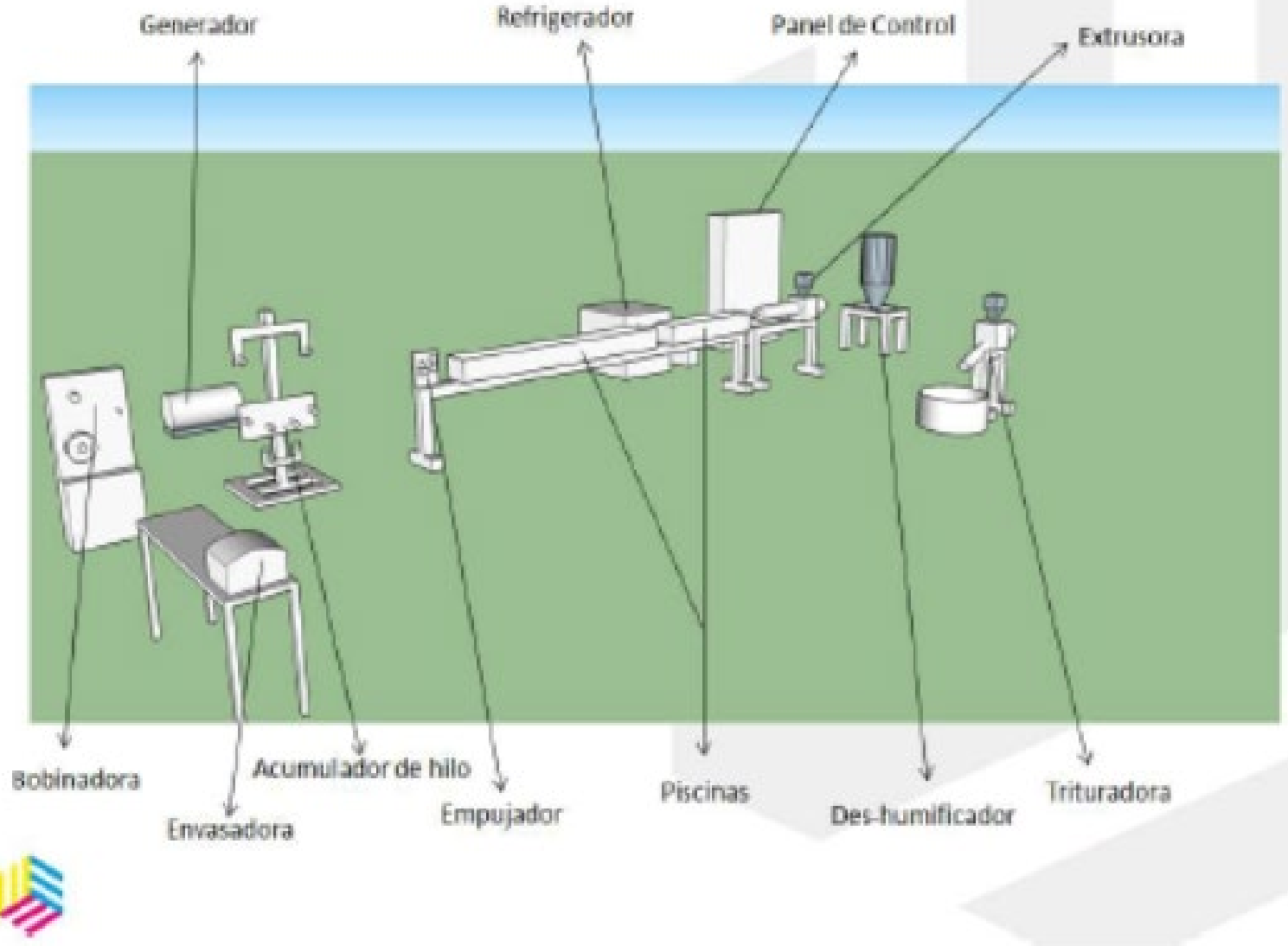
2 Esquema línea de producción
